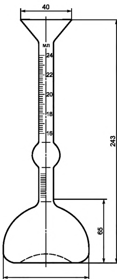
Рисунок 1 — Прибор Ле Шателье
