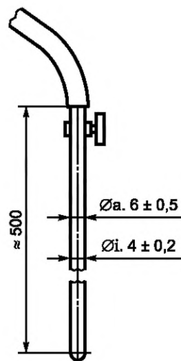
Рисунок 2 — Промывная трубка
