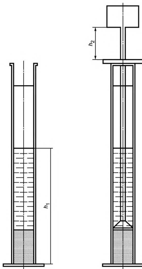
Рисунок 4 — Измерение высот h_1 и h_2
