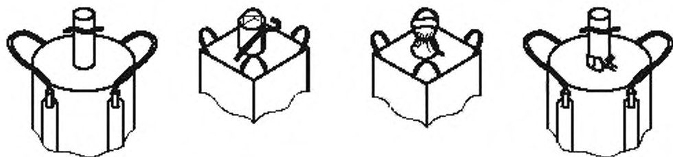
Рисунок Е.5 — Крышка с загрузочным рукавом
