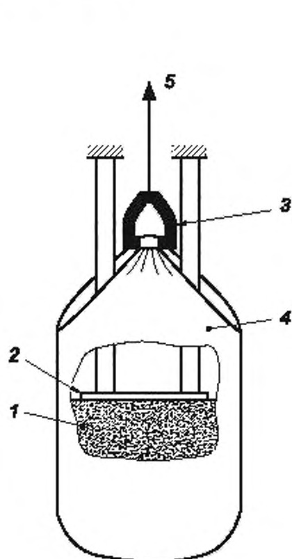
1 — наполнитель; 2 — нажимная плита; 3 — подвесная рама; 4 — МК; 5 — подъемный механизм
