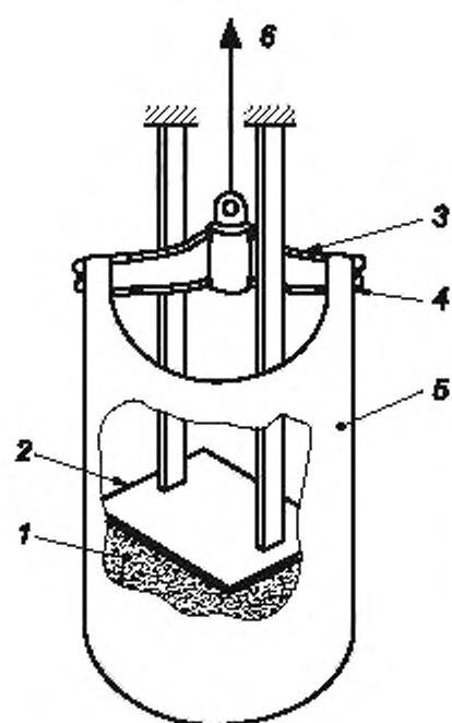
1 — наполнитель; 2 — нажимная плита; 3 — подвесная рама, 4 — устройство подъема МК, 5 — МК; 6 — подъемный механизм
