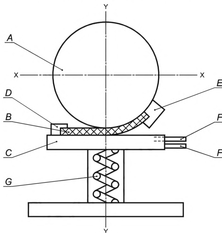
A — латунный ролик; B — испытуемая проба; C — платформа; D — зажим; E — зажим; F — подача воды; G — пружина
