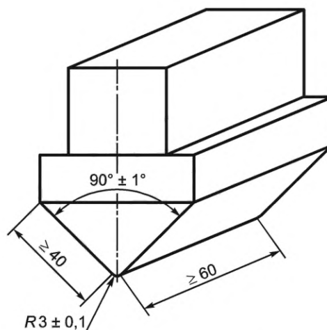
Рисунок 4 — Ударный боек
