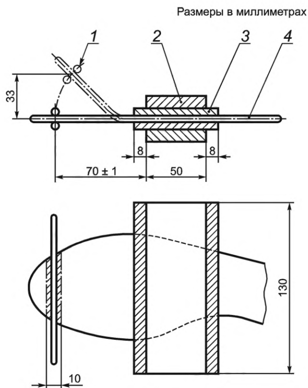
Рисунок 1 — Пример деталей подходящей конструкции аппаратуры для испытания на изгиб для неметаллических антипрокольных прокладок
