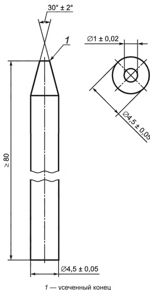
Рисунок 3 — Испытательный гвоздь для определения сопротивления проколу
