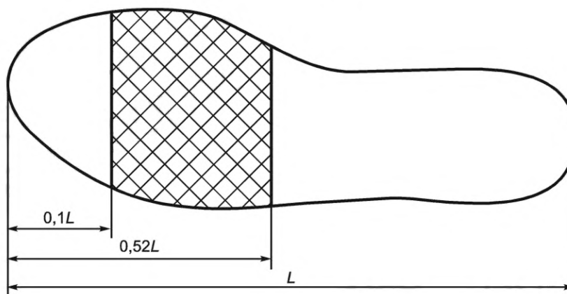
L — общая длина металлической прокладки
