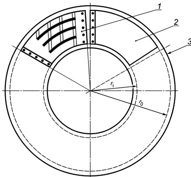
1 — гофрированный лепесток; 2 — верхний лепесток; 3 — пластина подшипника; r_i — внутренний радиус верхнего лепестка; r_o — наружный радиус верхнего лепестка
