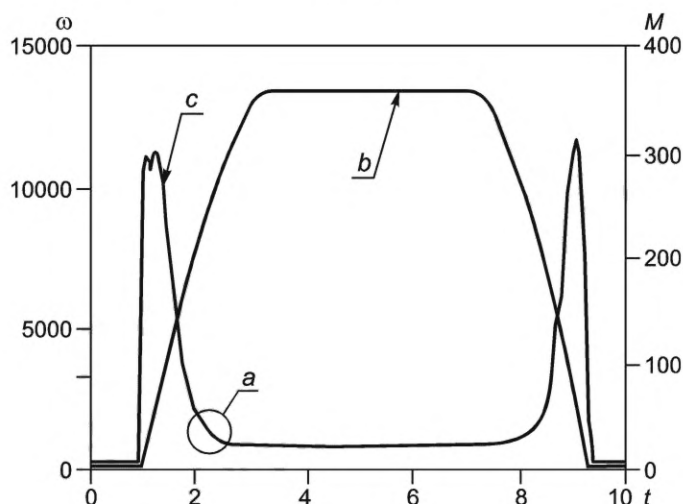
t — время в секундах; \omega — частота вращения мотора в оборотах в минуту; M — момент вращения в ньютон-миллиметрах; a — всплытие; b — кривая частоты вращения \omega ; c — кривая момента вращения M
