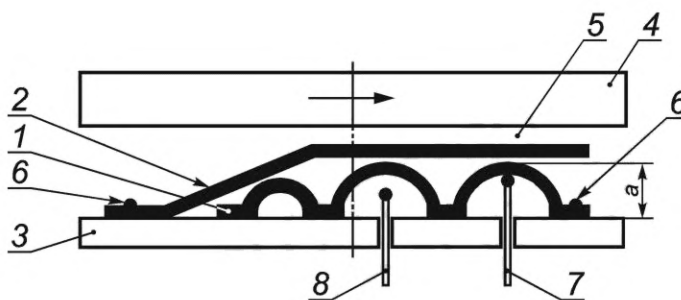
1 — гофрированный лепесток; 2 — верхний лепесток; 3 — пластина подшипника; 4 — ротор; 5 — воздушная пленка; 6 — точка сварки; 7 — термопара для измерения температуры поверхности верхнего лепестка; 8 — термопара для измерения температуры воздуха; a — высота гофрирования
