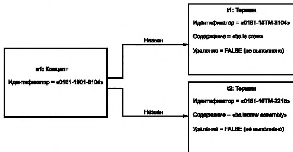
Рисунок D.2 — Состояние OTD после добавления неправильно написанного термина
