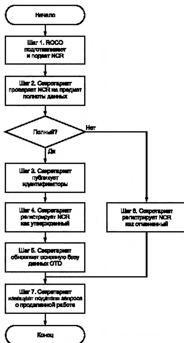
Рисунок 2 — Процедура добавления концепта
