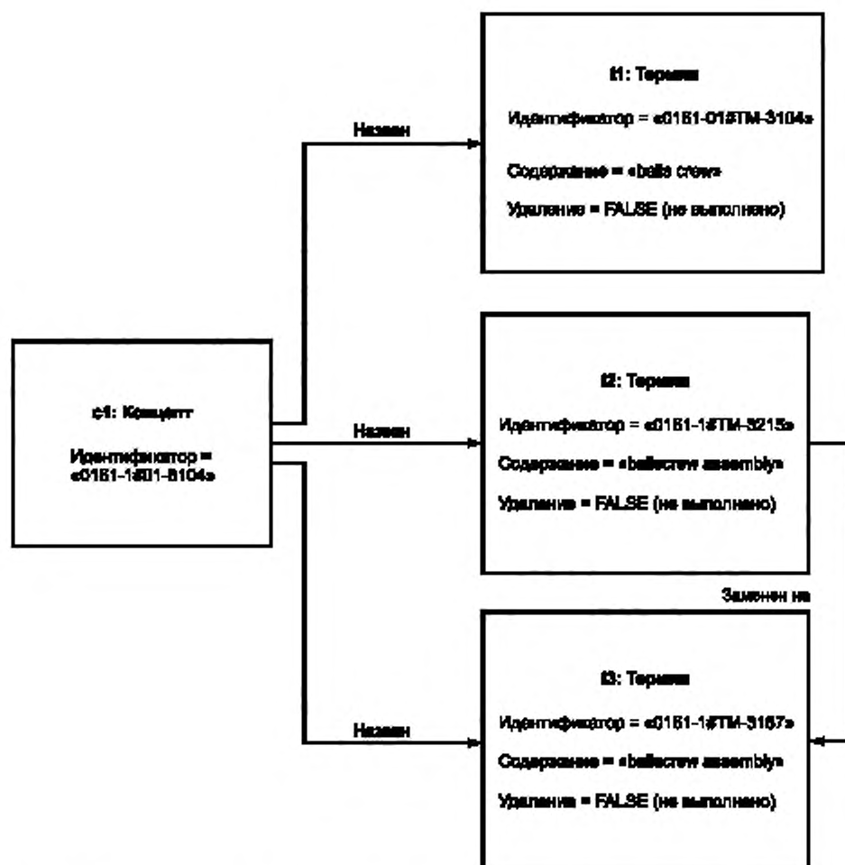
Рисунок D.3 — Состояние OTD после добавления нового термина, исправляющего ошибку предыдущего термина
