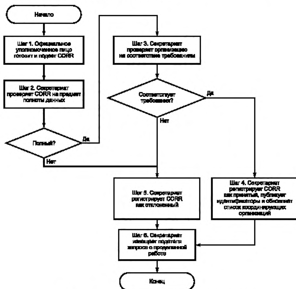
Рисунок 1 — Процедура регистрации координирующей организации
