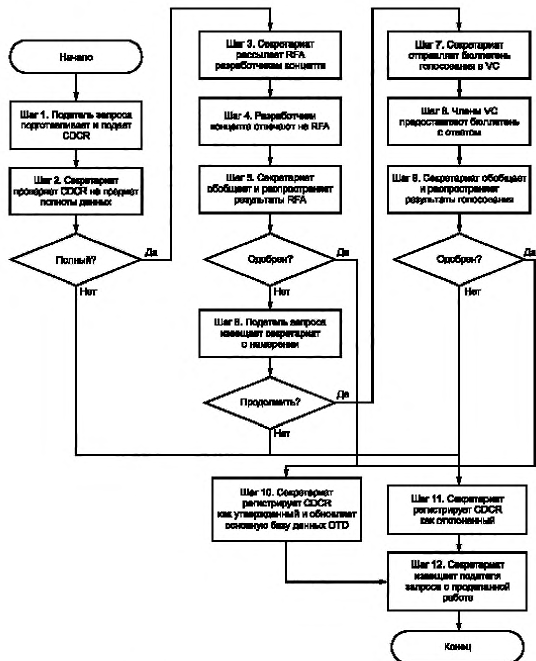
Рисунок 3 — Процедура изменения документации на концепт
