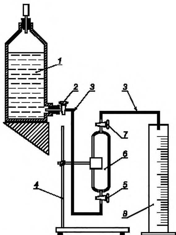
1 — склянка с тубусом (бутыл Вульфа); 2 — кран; 3 — соединительные шланги; 4 — штатив; 5, 7 — краны пипетки; 6 — пипетка; 8 — мерный цилиндр
