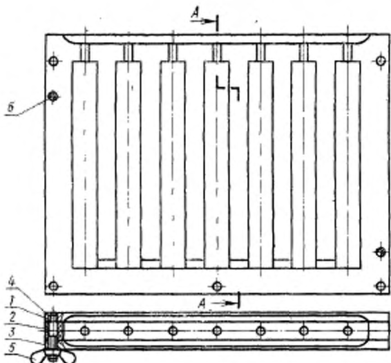
1, 3—наружные плиты; 2—вкладыш; 4—шпилька 7009—0266; 5—барашек М6; 6—штифт 51×18
