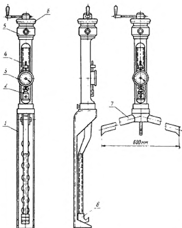
1—упор; 2—пружина; 3—индикатор; 4—корпус; 5—шарнир; 6—линь с ручкой; 7—собственная база; 8—крюк
