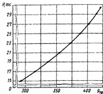
Градуировочная характеристика прибора ПРДУ
