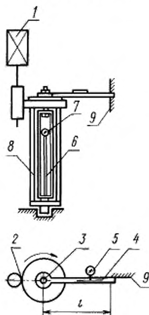
1 — электродвигатель; 2 — редуктор; 3 — проверяемый болт; 4 — динамометрический ключ; 5 — индикатор динамометрического ключа; 6 — динамометр для измерения усилия натяжения болта; 7 — индикатор динамометра; 8 — корпус прибора; 9 — упор ключа
