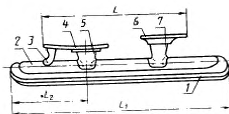
Конек беговой (цельнометаллический)
