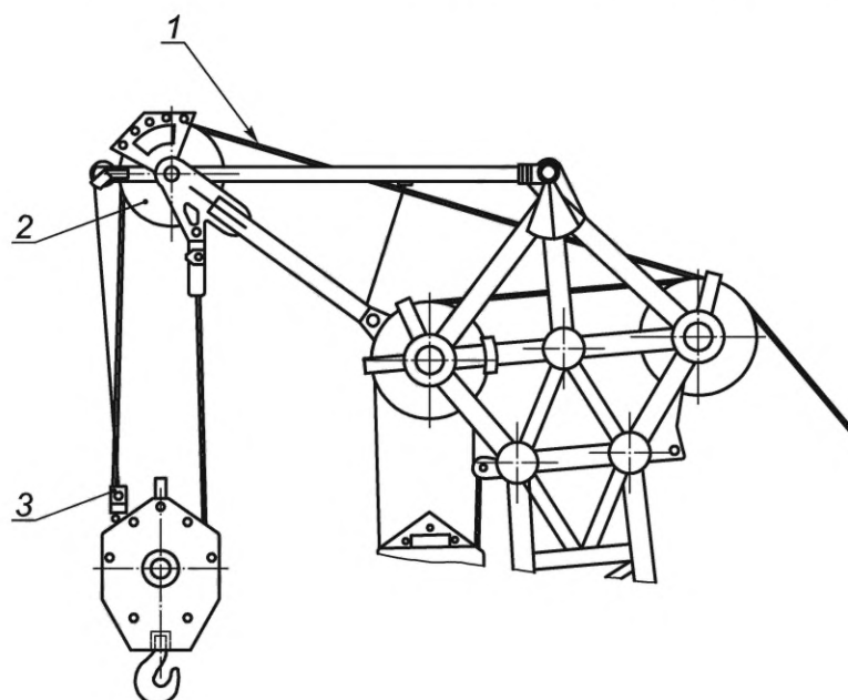
1 — рама в сборе; 2 — шкив; 3 — верхний концевой выключатель
