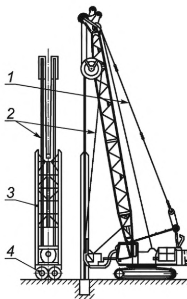
1 — полиспаст для гидравлических рукавов и рукавов подвески; 2 — цилиндр подачи; 3 — направляющая рама; 4 — колесо резака
