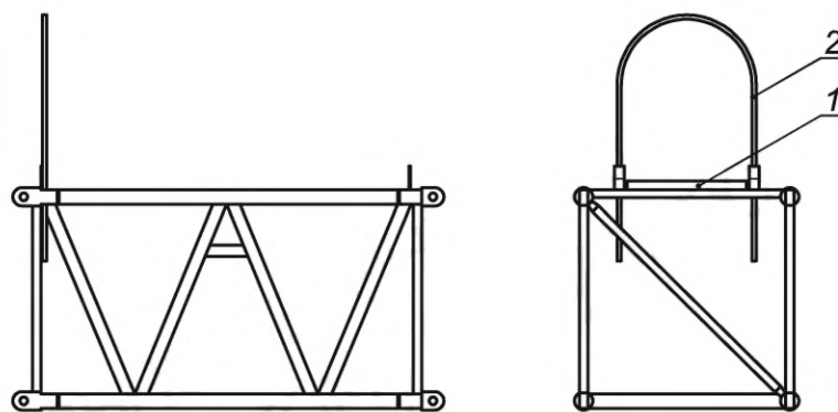
1 — защита каната; 2 — корзина каната
