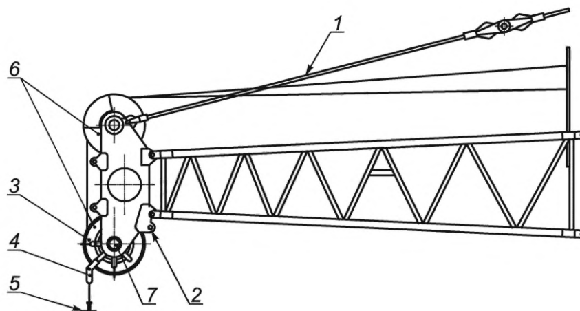
1 — канат подвески стрелы; 2 — точка фиксации каната для системы запасовки каната; 3 — защита каната; 4 — верхний концевой выключатель
