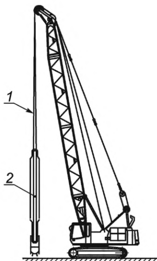
Рисунок 28 — Оборудование для резки стен
