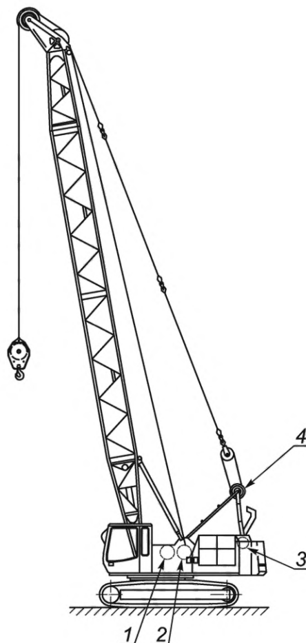
Рисунок 14 — Расположение лебедки и шкива
