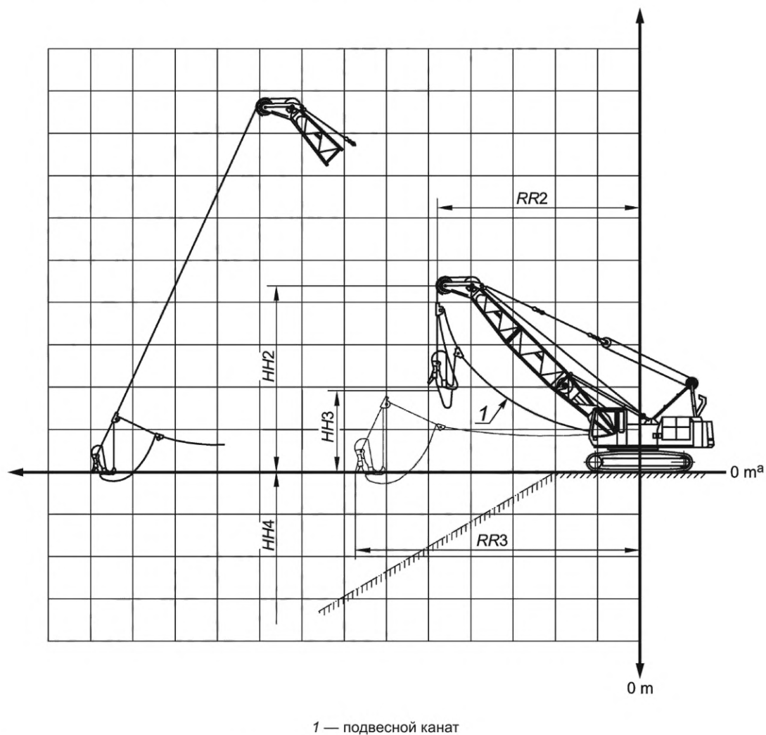
Рисунок 7 — Размерные характеристики драглайна
