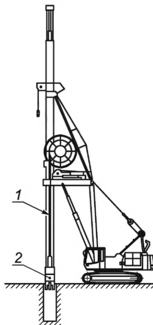
1 — ведущая штанга; 2 — диафрагменный стеновой захват
