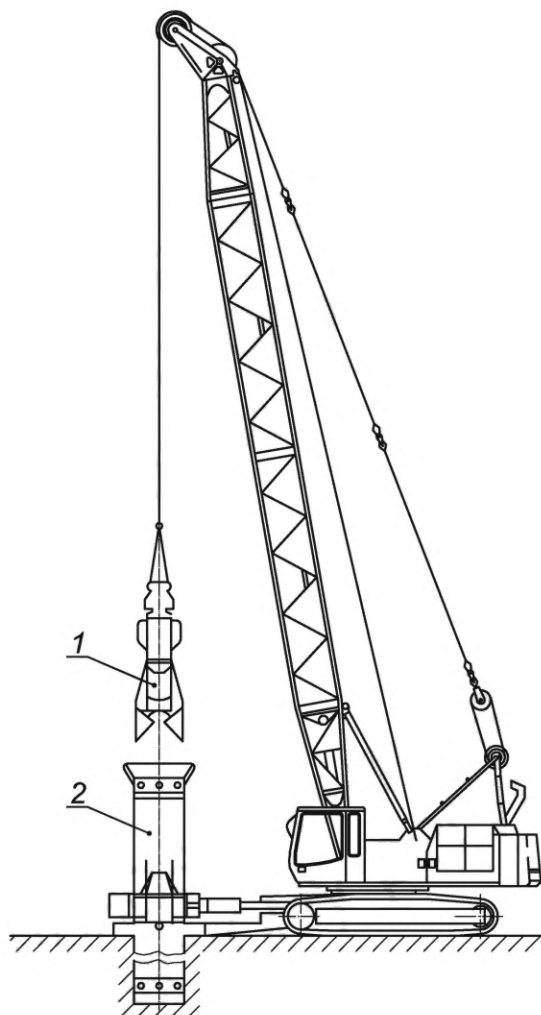
Рисунок 25 — Обсадной вибратор
