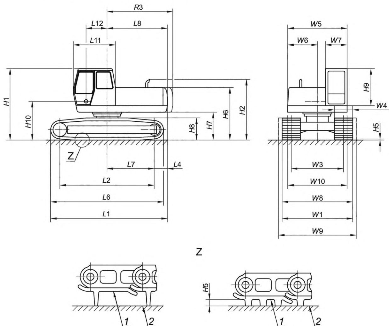
Рисунок 3 — Размерные характеристики базовой машины. Гусеничный экскаватор
