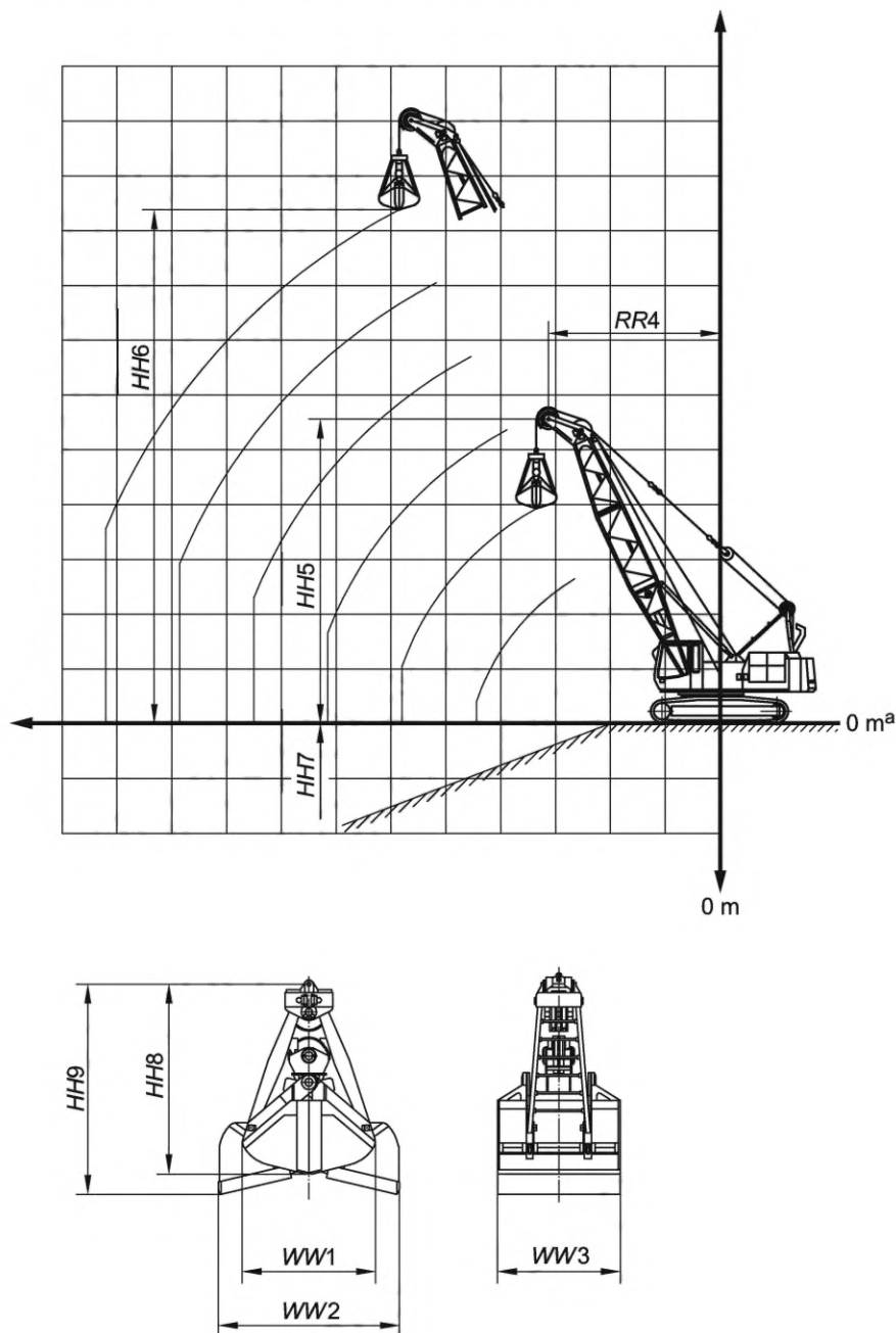
Рисунок 8 — Размерные характеристики захвата/грейфера и его оборудования
