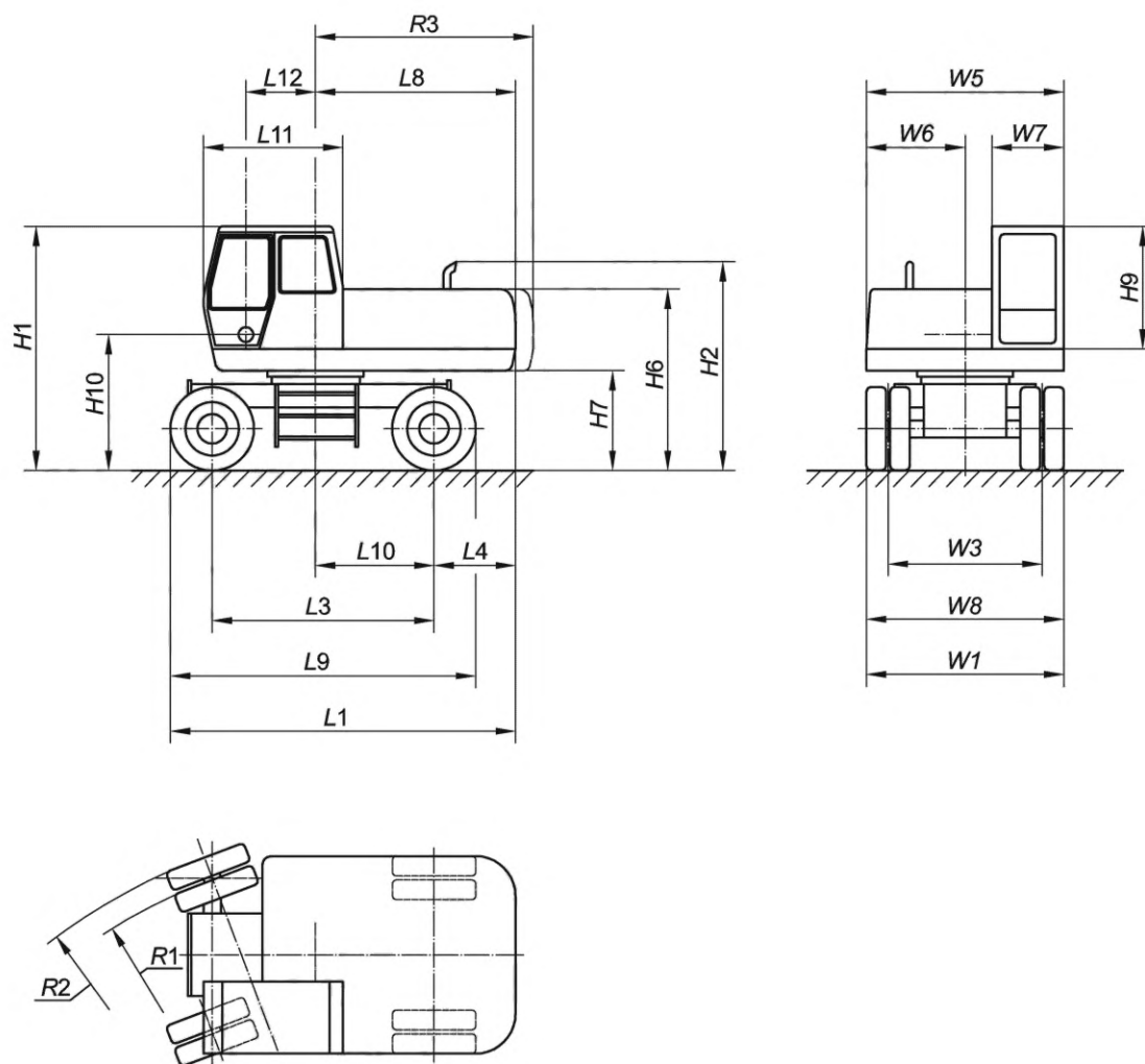
Рисунок 4 — Размерные характеристики базовой машины. Колесный экскаватор
