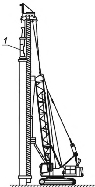
Рисунок 27 — Сваеабивное оборудование
