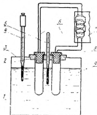
1 — теплоноситель — вода, 2 — крышка термостата; 3 — термостат; 4 — контактный термометр; 5 — ртутный термометр; 6 — термопара; 7 — потенциометр; 8 — вкладыш из фторопласта, 9 — наружная пробирка (см. черт. 2)
