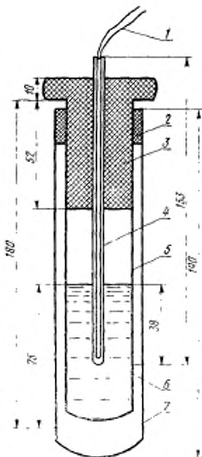
1—термopapa; 2—кольцо из пенополистирола; 3—вкладыш из фторопласта; 4—чекол; 5—внутренняя пробирка; 6—смола; 7—внешняя пробирка. Черт. 2
