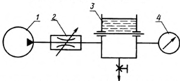
Установка для определения герметичности
