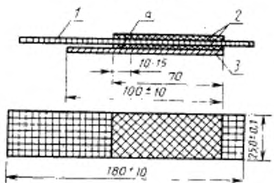
Схема образца
