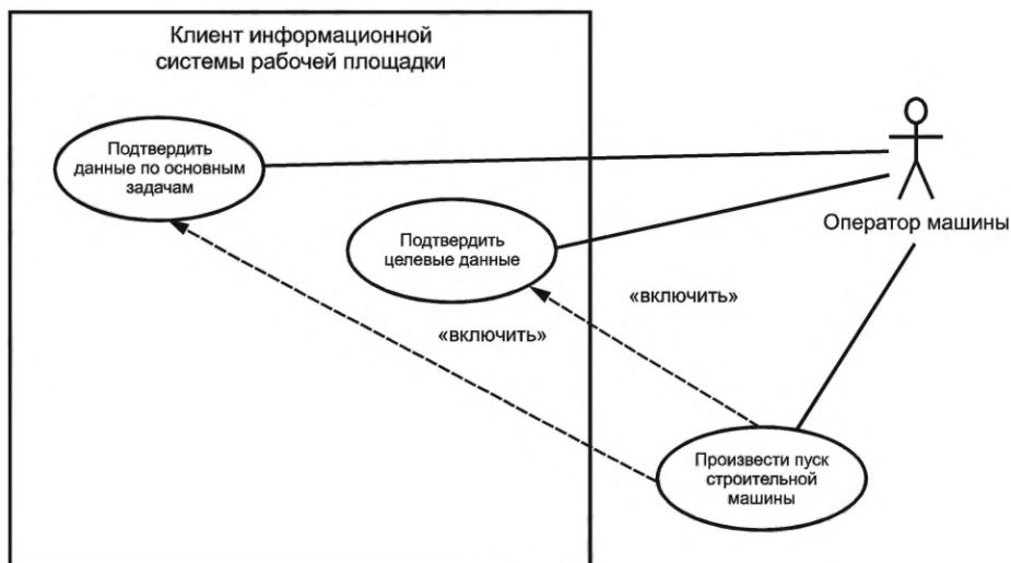
Рисунок D.4 — Диаграмма варианта использования. Услуга по поддержанию машинных операций
