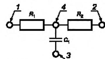
Рисунок В.1 — Составная мера активного сопротивления и емкости
