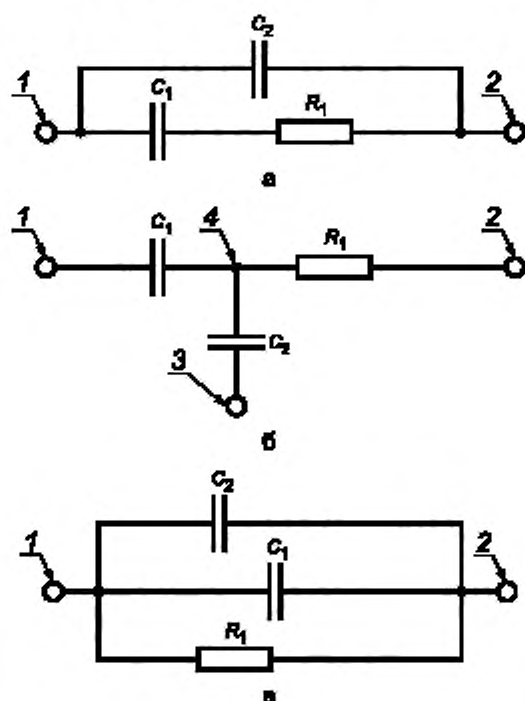
Рисунок В.3 — Составные меры тангенса угла потерь
