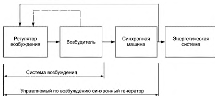
Рисунок 1 — Структура управляемого по возбуждению синхронного генератора
