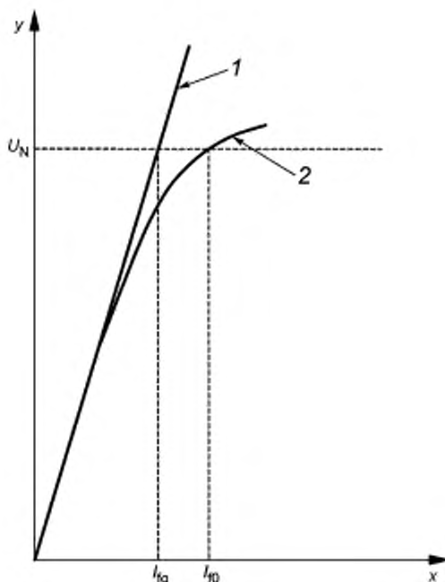
y — ось напряжений U на выводах машины ( U_N — номинальное напряжение); x — ось токов возбуждения I_f ; 1 — линейная характеристика воздушного зазора; 2 — характеристика холостого хода
