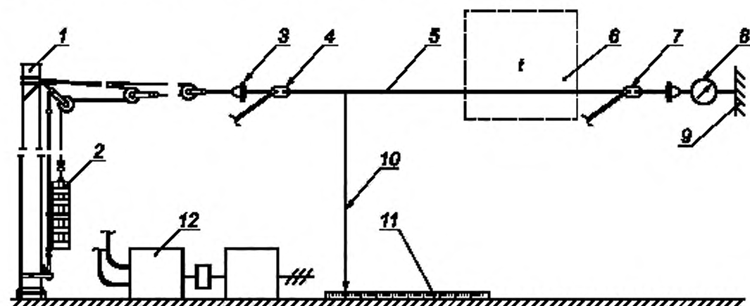
1 — опора; 2 — грузокompенсатор; 3 — изолятор; 4 — питающие зажимы; 5 — испытуемый кусок провода; 6 — место замера температуры ( t ); 7 — динамометр; 8 — жесткий крепеж провода; 9 — отвес; 10 — линейка; 12 — источник питания
