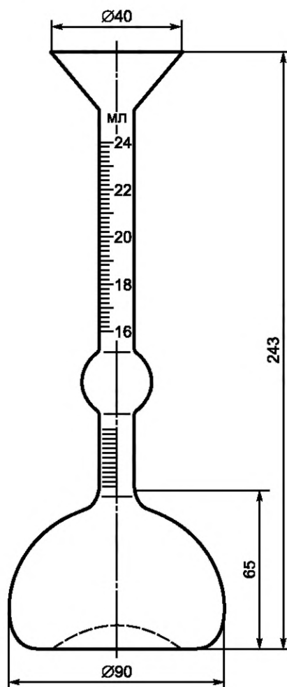
Рисунок 1 — Прибор Ле-Шателье
