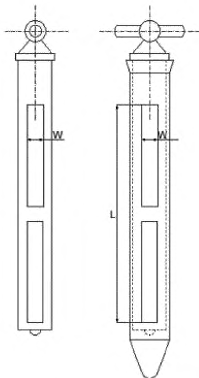
Рисунок 1 — Схема пробоотборника
