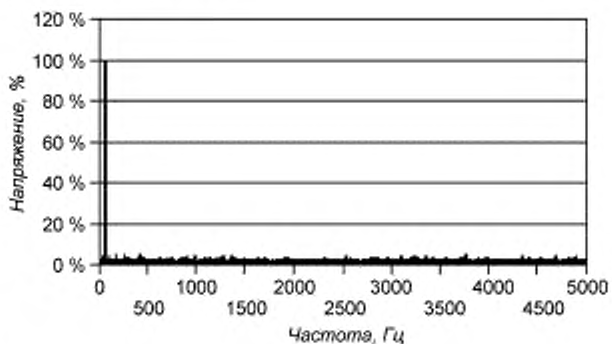
Спектр частот напряжения на выходе преобразователя — инвертора напряжения типа В, f_1 = 50 Гц, f_{s\text{cp}} = 4,5 кГц
