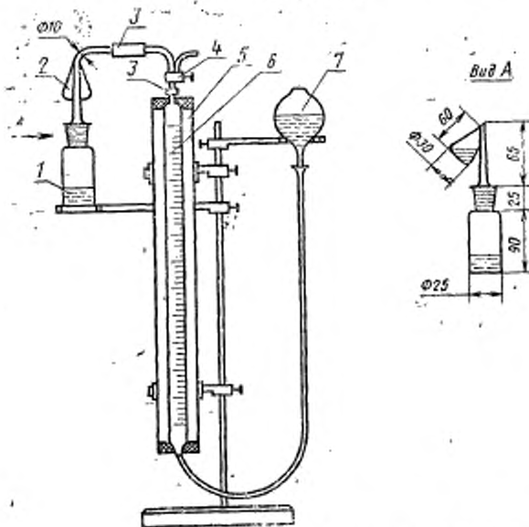
1—реакционная пробирка; 2—боковой карман; 3—вакуумный надув; 4—кран трехходовой; 5—водяной кожух; 6—бюретка; 7—уравнительный сосуд.
