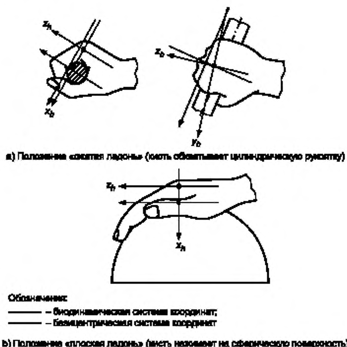
Рисунок 1 — Направления измерений
