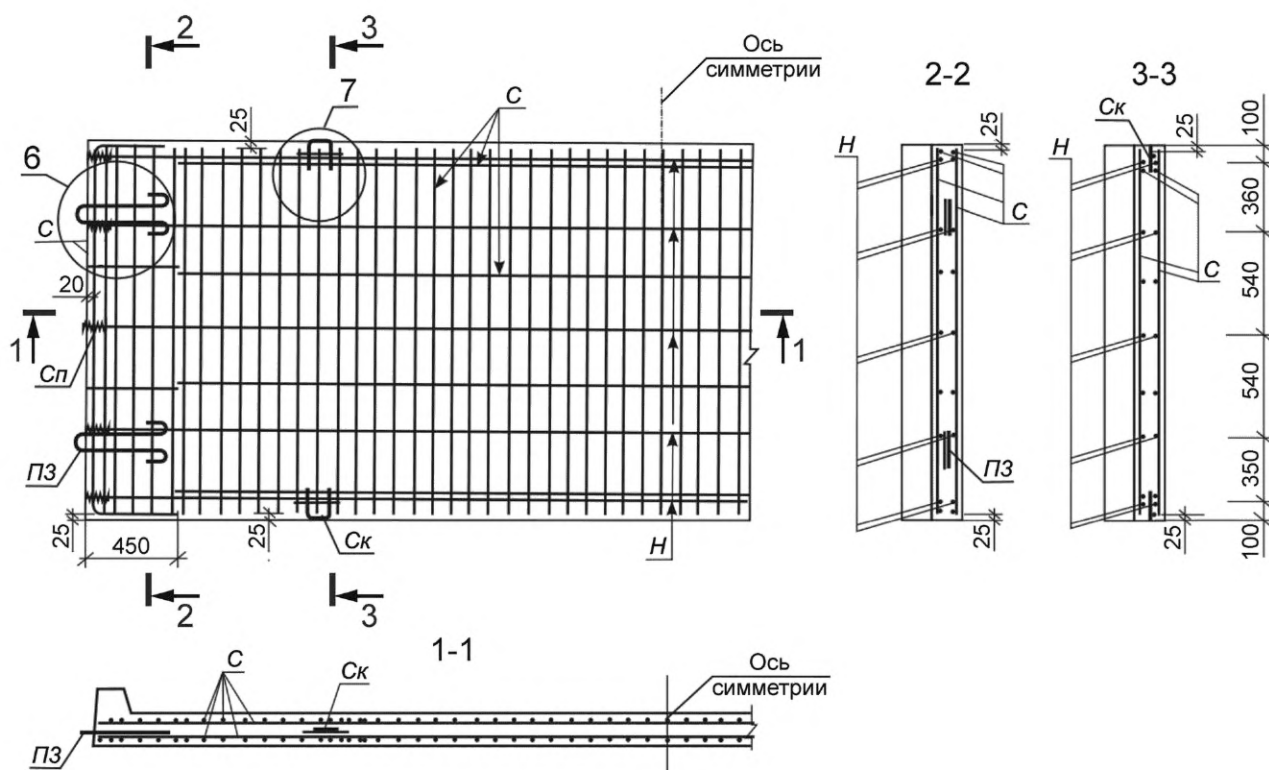
Рисунок Б.4 — Схема армирования плиты ПБ55.20
