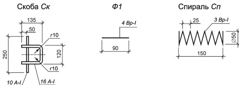
Рисунок Г.3 — Скоба Ск, спираль Сп, фиксатор Ф1
