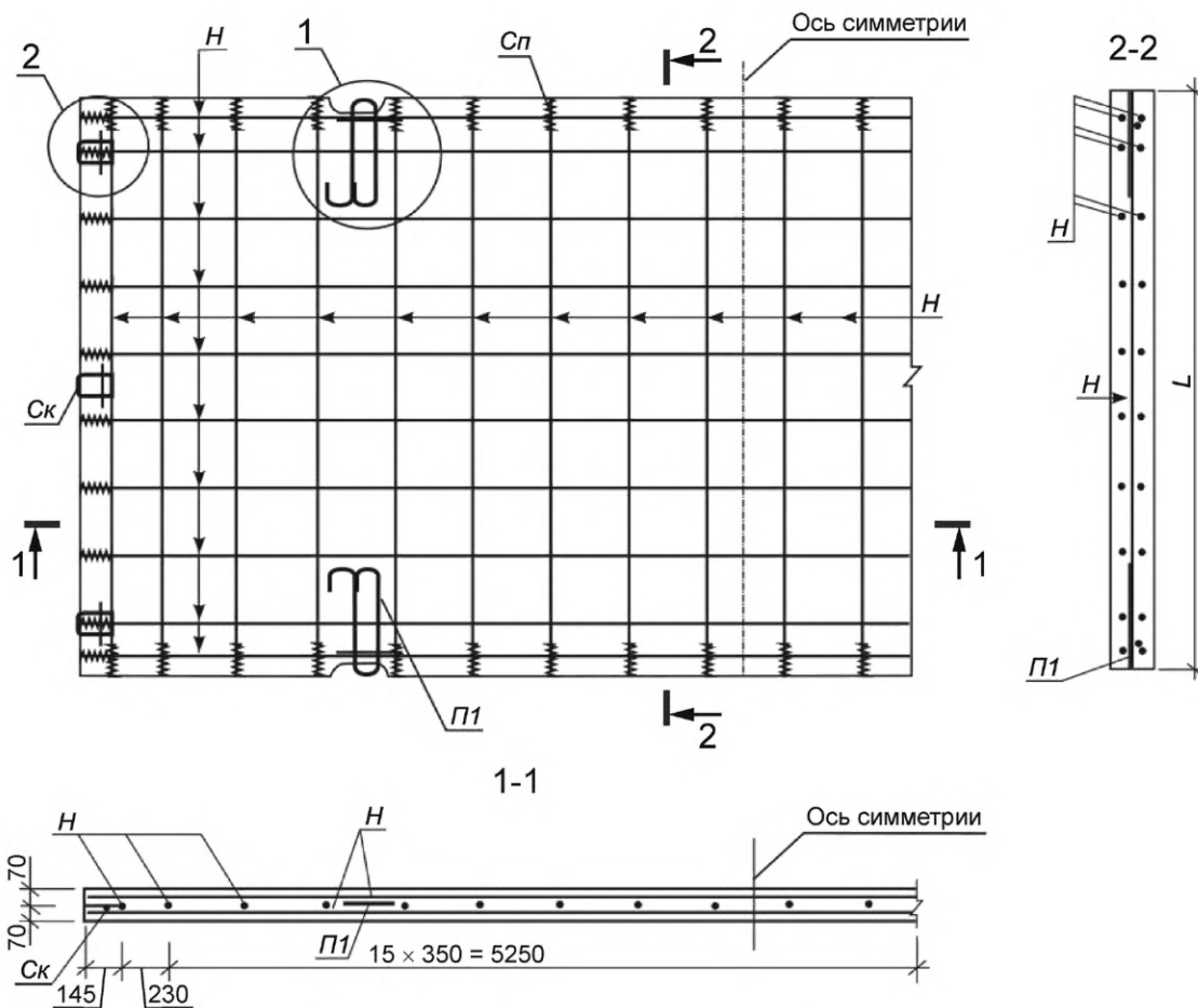
Рисунок Б.1 — Схемы армирования плит П60.38, П60.35, П60.30
