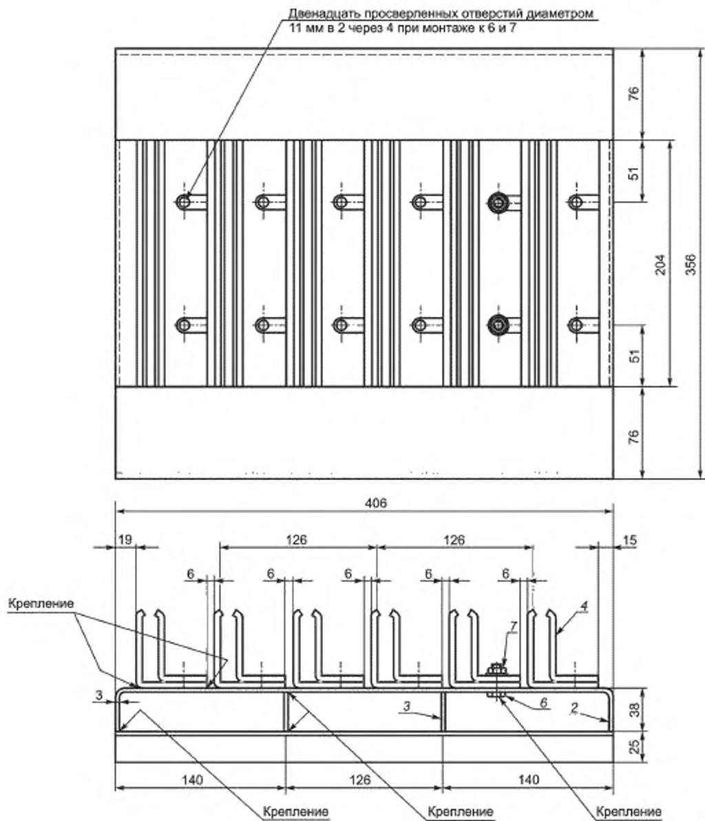
Рисунок А.1 — Типичный монтаж паза
