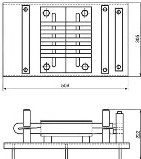
Рисунок А.3 — Типовое приспособление для испытания катушки ротора постоянным током
