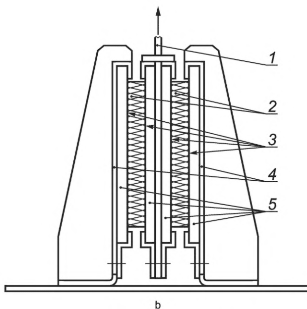
Рисунок 1 — Схема устройства с одним образцом
