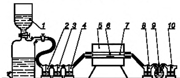
Схема установки для определения углерода
