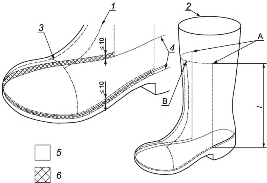
1 — центральная линия обуви; 2 — верхняя часть верха; 3 — задний край защитного носка; 4 — линия кромки; 5 — защитная область; 6 — дополнительная защитная область для обуви уровня защиты 3
