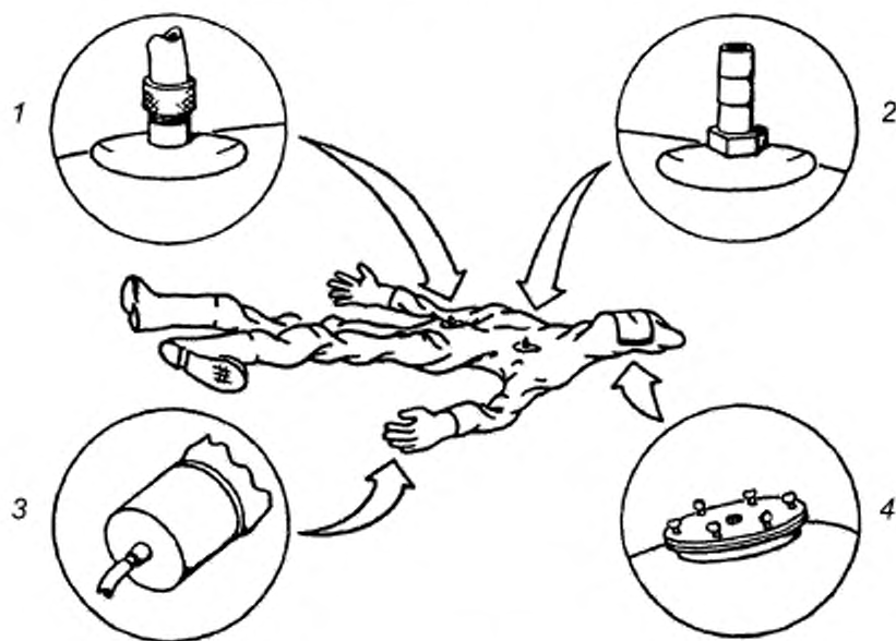
1 — соединительный элемент или разъем для подключения линии сжатого воздуха; 2 — адаптер для подключения к вентиляционному клапану; 3 — адаптер для подключения к соединению костюма с перчатками; 4 — адаптер для подключения к соединению костюма с лицевой частью
