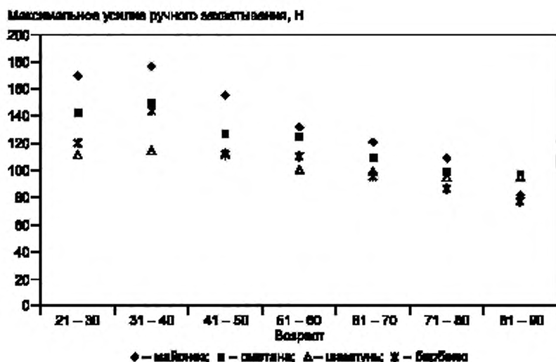
Рисунок С.5 — Максимальное усилие ручного захватывания в зависимости от возраста для четырех различных типов продукции
