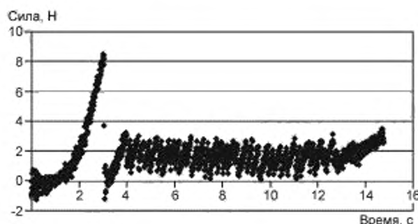
Рисунок С.7 — Типичная прочность соединения отслаиваемого покрытия для упаковки с крышкой
