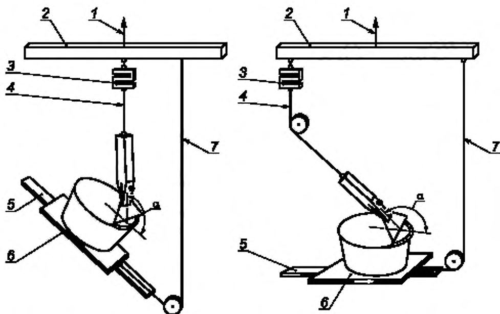
1 — направление движения траверсы; 2 — траверса; 3 — силоизмеритель; 4 — соединение силоизмерителя с зажимом. 5 — направляющая; 6 — ползун; 7 — соединение ползуна с траверсой, а — угол наклона при отслаивании
