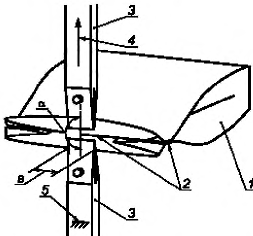
1 — пакет с боковой складкой; 2 — сварной шов; 3 — зажимы для пленочного покрытия. 4 — направление движения, 5 — фиксация; В — ширина зажима для пленочного покрытия; α — угол при разрывании
