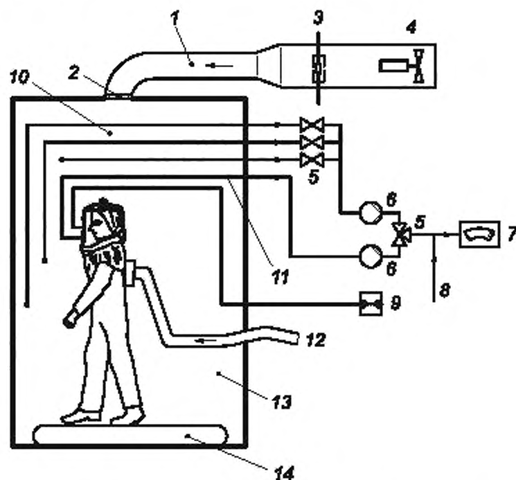
1 -- труба; 2 -- заслонка; 3 -- распределитель воздушного потока; 4 -- вентилятор; 5 -- переключающий клапан; 6 -- насос; 7 -- анализатор \text{SF}_6 ; 8 -- дополнительная подача воздуха; 9 -- манометр; 10 -- пробоотборник в камере; 11 -- пробоотборник в дыхательной зоне; 12 -- воздух для дыхания; 13 -- камера; 14 -- беговая дорожка
