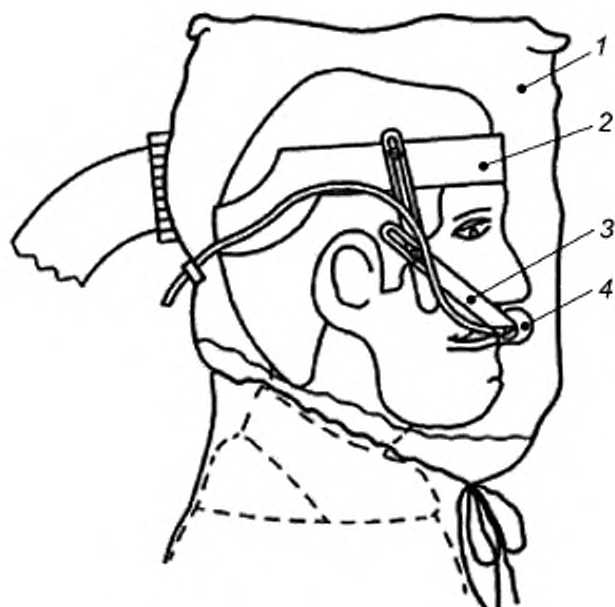
1 — капюшон; 2 — оголовье; 3 — регулируемый держатель пробоотборника; 4 — пробоотборник
