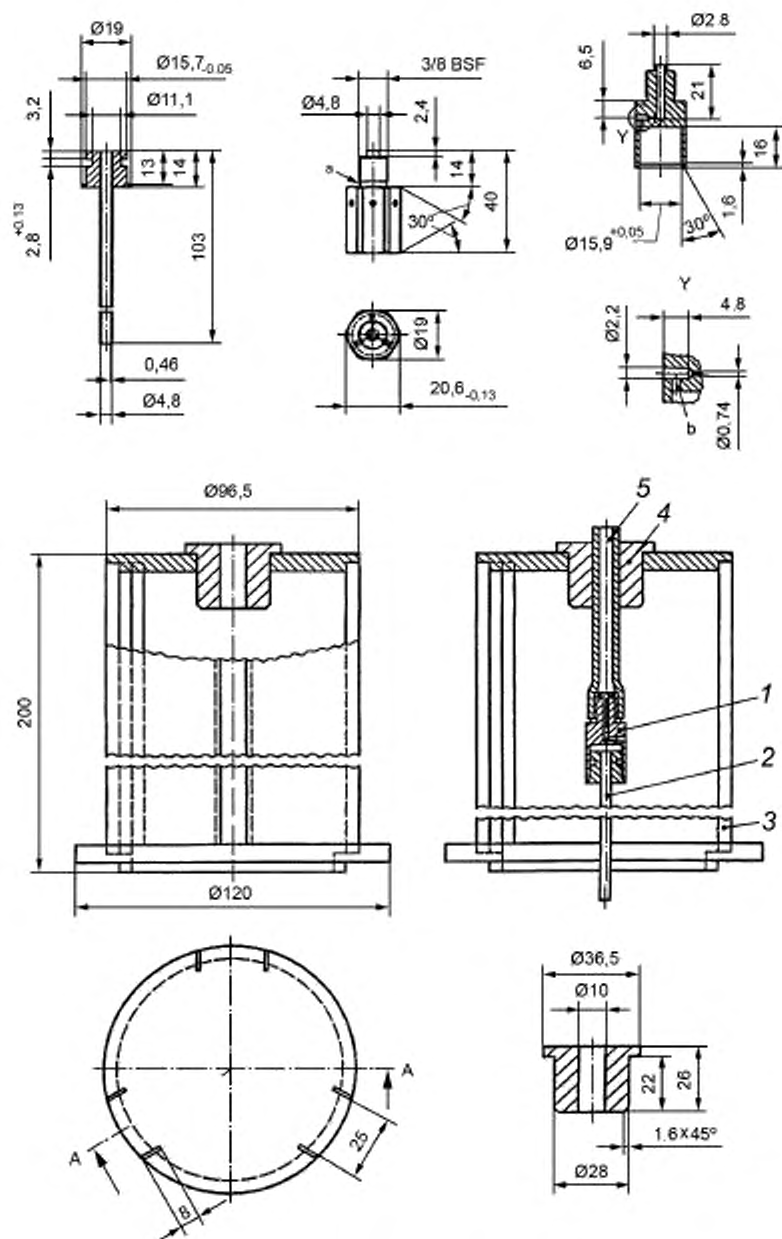
Рисунок 3 — Конструкция распылителя
