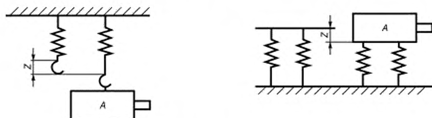
A — машина; Z — упругая деформация крепления
