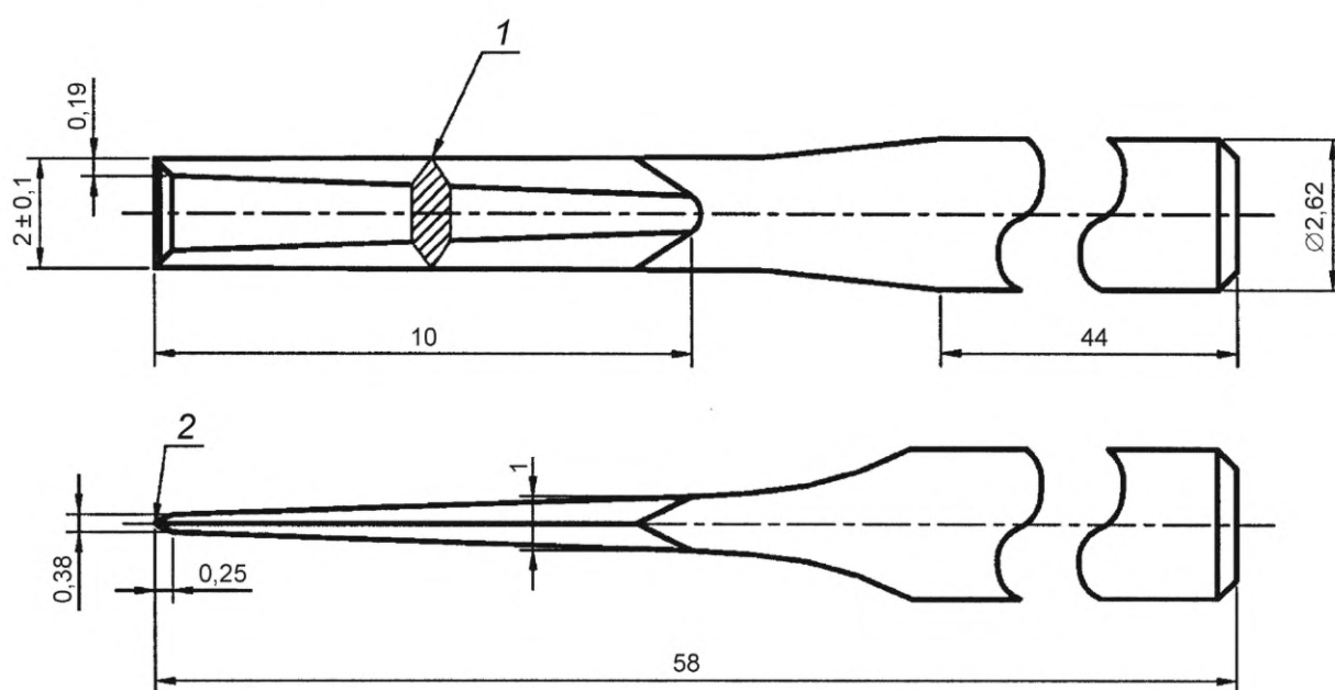
1 — острый конец с прямыми углами на обеих сторонах лезвия от конуса до острия; 2 — острый конец
