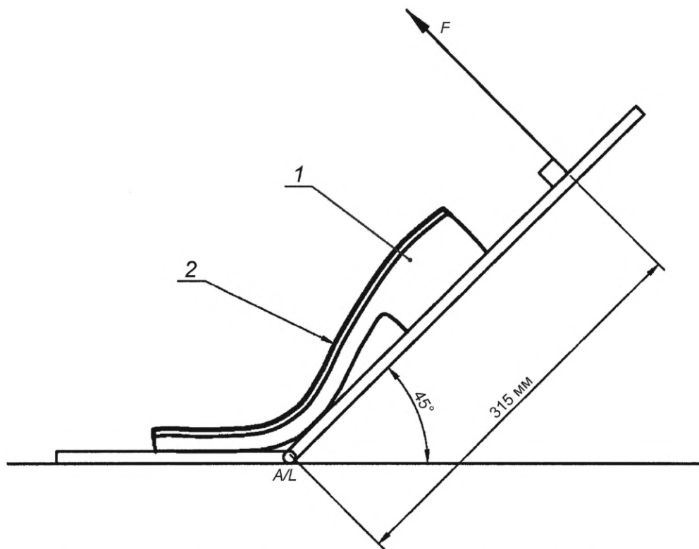
Рисунок 1 — Устройство измерения жесткости подошвы при растяжении
