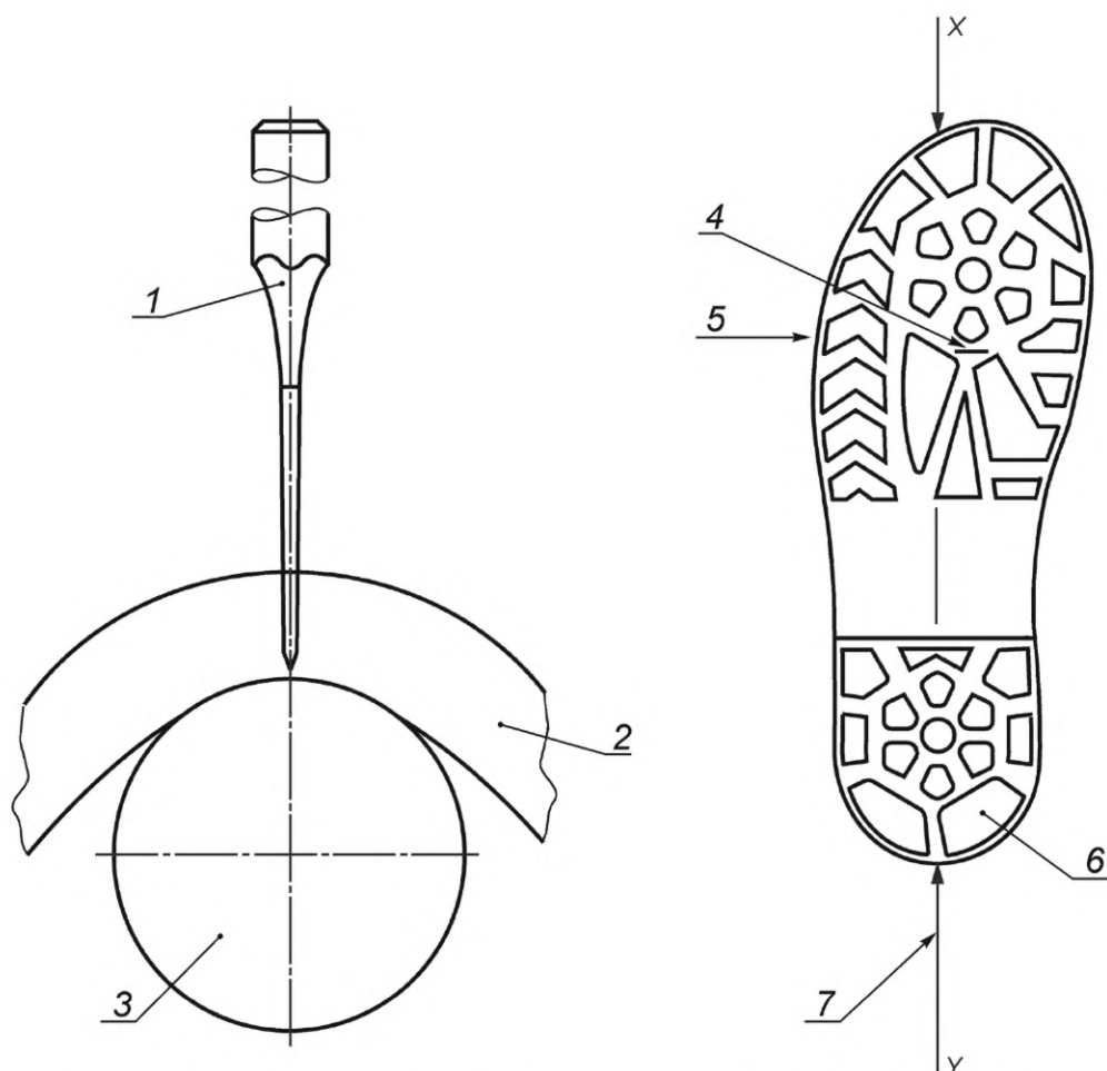
1 — режущий инструмент; 2 — испытуемый образец; 3 — сердечник испытательной машины; 4 — единственный надрез параллельно линии максимального давления; 5 — линия максимального давления (деформации) AC; 6 — протектор на подошве (рельефный рисунок на ходовой поверхности подошвы); 7 — продольная ось XY
