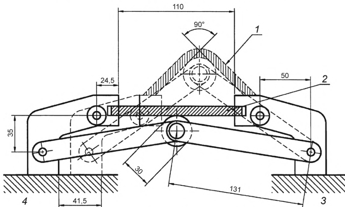
Рисунок 1 — Устройство измерения жесткости подошвы при растяжении
