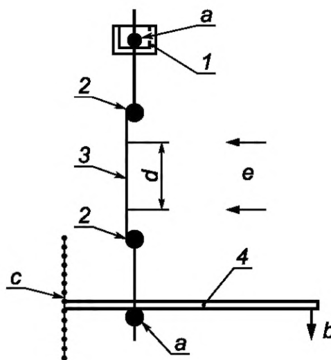
1 — жесткая рамка; 2 — зажим для испытуемого образца; 3 — испытуемый образец; 4 — грузоподъемник; a — сферическая насадка; b — нагрузка; c — регулируемый центр вращения для постоянной нагрузки; d — номинальная длина; e — удаленное измерение с помощью экстензометра
