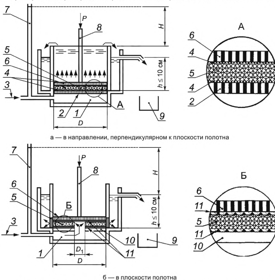
1 — фильтрационная камера внутренним диаметром D ; 2 — перфорированный диск; 3 — устройство для подачи воды; 4 — сетка; 5 — проба геосинтетического материала; 6 — перфорированный штамп; 7 — пьезометрическая трубка; 8 — устройство для передачи давления ( P ) на пробу; 9 — емкость для сбора и измерения объема воды; 10 — диск с отверстием диаметром D_1 для подачи воды; 11 — резиновые прокладки; H — значение напора; h — уровень воды на выходе из прибора
