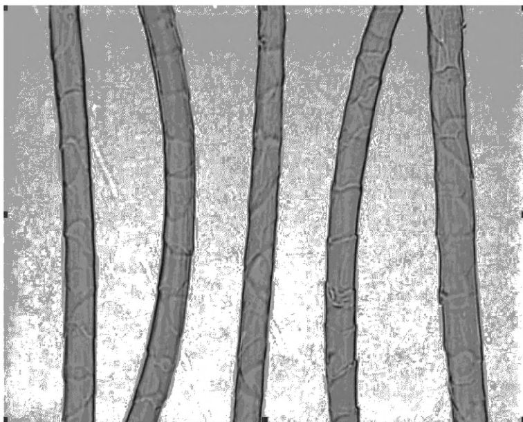
Рисунок С.26 — Изображение волокон с неравномерным расстоянием между чешуйками
