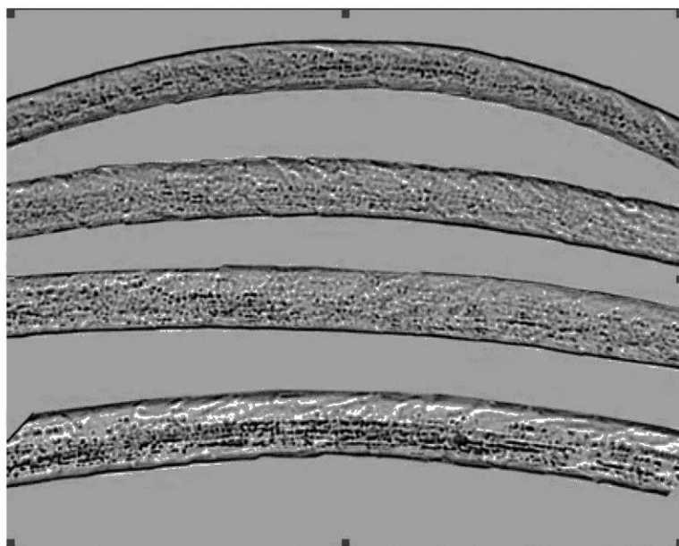
Рисунок С.47 — Изображение волокон обесцвеченной верблюжьей шерсти с не полностью удаленным пигментом
