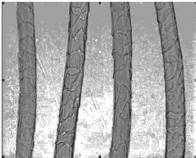
Рисунок С.33 — Изображение волокон с чешуйками неправильной формы на неровной поверхности волокна с углублениями, показанными на стволе волокна
