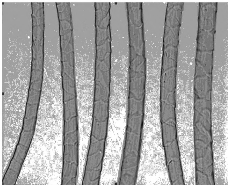
Рисунок С.29 — Изображение волокон с чешуйками с непостоянным кольцевидным расположением и тонкими чешуйками с повышенной частотой
