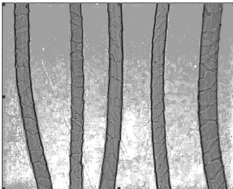
Рисунок С.28 — Изображение волокон с чешуйками с непостоянным кольцевидным расположением, расположенными под большим углом
