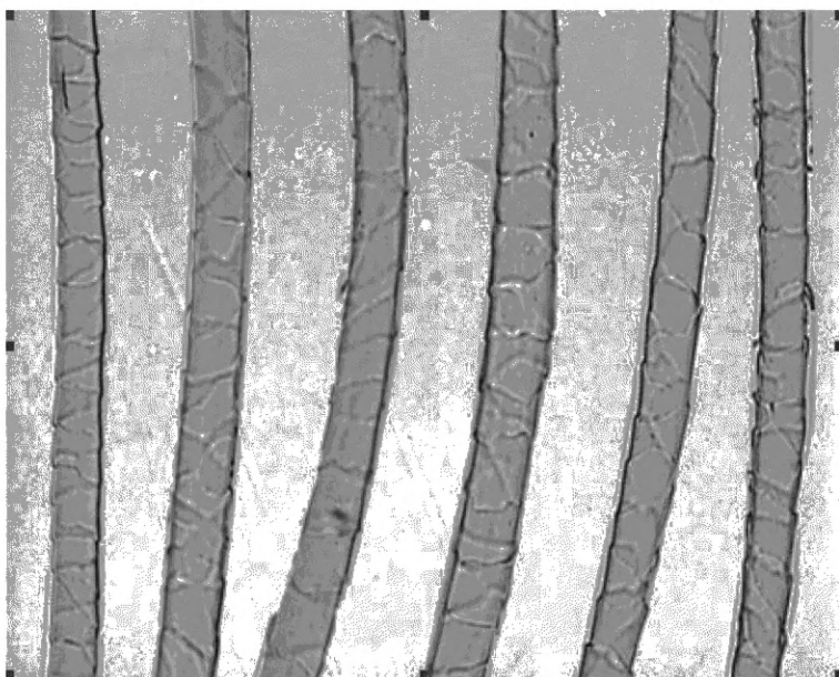
Рисунок С.23 — Изображение волокон с тонкими чешуйками, частота чешуек высокая
