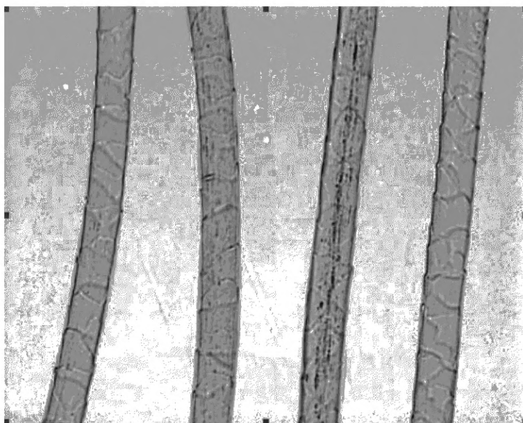
Рисунок С.21 — Изображение волокон, высота чешуек которых незначительно увеличена
