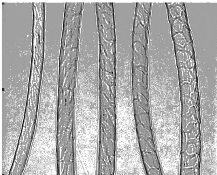
Рисунок С.45 — Изображение волокон обесцвеченной верблюжьей шерсти. Достаточно большая высота чешуек и существенное непостоянство расположения чешуек, подобные характерным для овечьей шерсти
