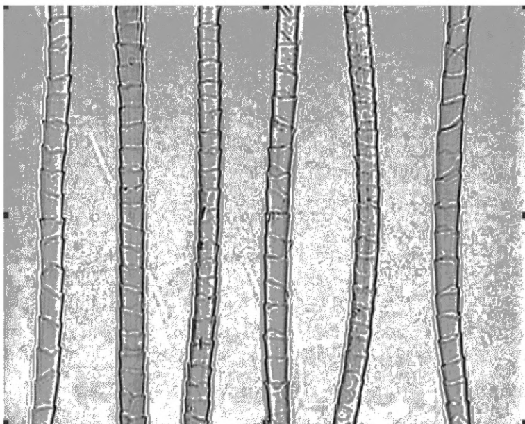
Рисунок С.11 — Изображение волокон с чешуйками венчиковидной формы с очень высокой частотой, имеющих характеристики тонкой овечьей шерсти
