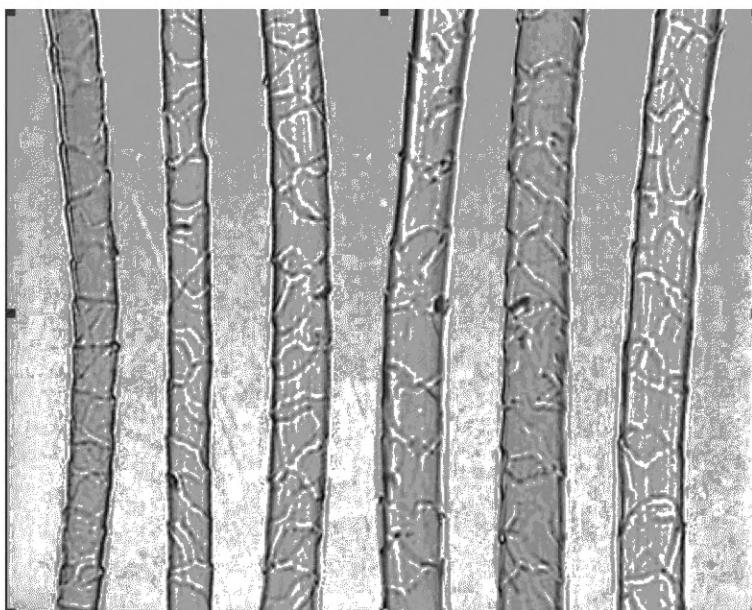
Рисунок С.14 — Изображение волокон, расположение чешуек которых не повторяется, поверхность волокон не гладкая, что является проявлением характеристик овечьей шерсти происхождением из Китая
