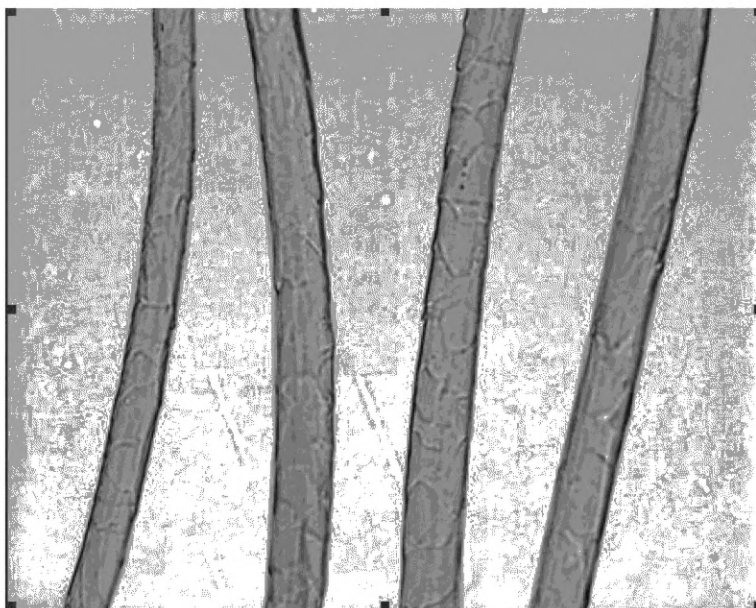
Рисунок С.27 — Изображение волокон, чешуйки которых неотчетливо видны и вызывают сомнение
