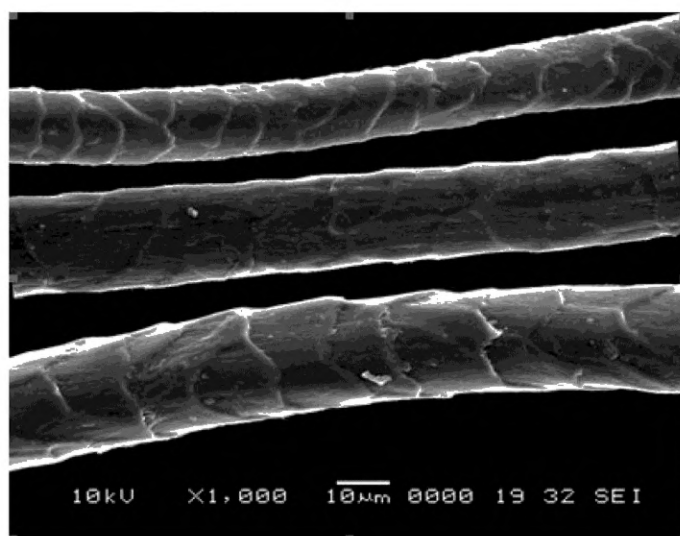
Рисунок В.64 — Изображение волокон безусадочной шерсти
