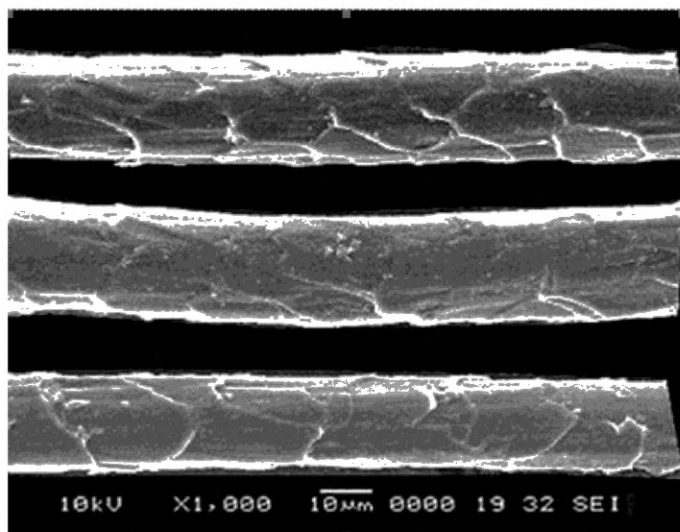
Рисунок В.59 — Изображение волокон с «размытыми» чешуйками
