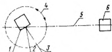
1—рентгеновская трубка; 2—действительное фокусное пятно рентгеновской трубки; 3—ось рабочего пучка рентгеновского излучения; 4—направление вращения рентгеновской трубки; 5—оптическая ось блока детектирования; 6—блок детектирования
