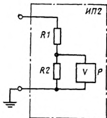
R1, R2 —резисторы делителя; P —вольтметр
