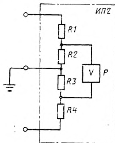
R1 \dots R4 —резисторы делителя; P —вольтметр
