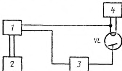
1 — управляемый источник напряжения свч — 1000 В; 2 — устройство задания длительности прохождения тока рентгеновской трубки; 3 — измеритель количества электричества; 4 — источник питания накала; VL — рентгеновская трубка
