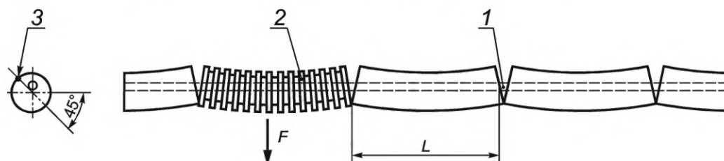
Рисунок 2 — Схема расположения стойки при проведении испытаний
