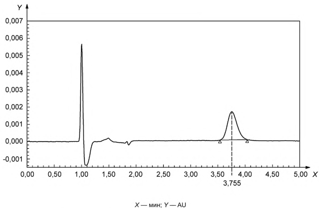
Рисунок В.1 — Хроматограмма, полученная для одного образца, содержащего 3,9 мг/кг Cr(VI)
