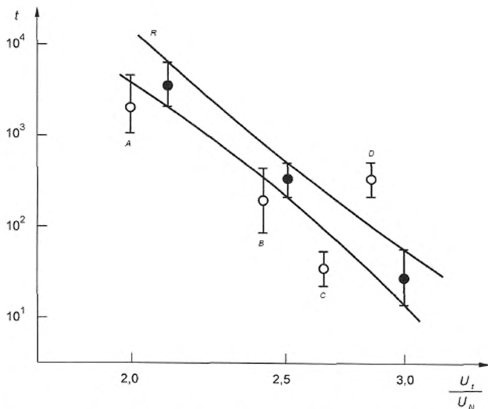
R — данные старения эталонной системы изоляции ( R ) с демонстрацией 90 % доверительного интервала; A — данные старения для испытуемой системы A (отказ в аттестации); B — данные старения для испытуемой системы B (успешная аттестация); C — данные старения для испытуемой системы C (отказ в аттестации); D — данные старения для испытуемой системы D (успешная аттестация); t — время в часах; U_t/U_N — отношение испытательного напряжения к номинальному
