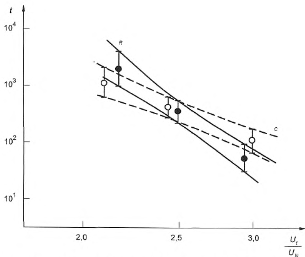
R — данные старения эталонной системы изоляции ( R ) с демонстрацией 90 % доверительного интервала; C — данные старения испытуемой системы изоляции ( C ) с демонстрацией 90 % доверительного интервала; t — время в часах; U_t/U_N — отношение испытательного напряжения к номинальному
