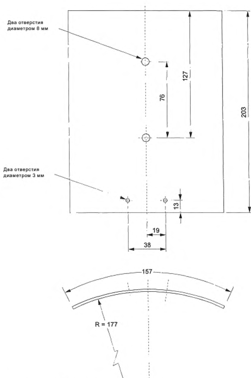
Рисунок В.8 — Производственный чертеж модели рамы для измерения обмотки
