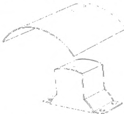
Рисунок В.1 — Испытательная арматура для нешаблонной обмотки
