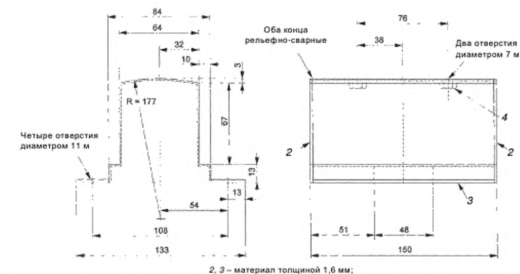
Рисунок В.7 — Производственный чертеж модели полюсного сердечника для измерения намотанной обмотки на испытательной арматуре
