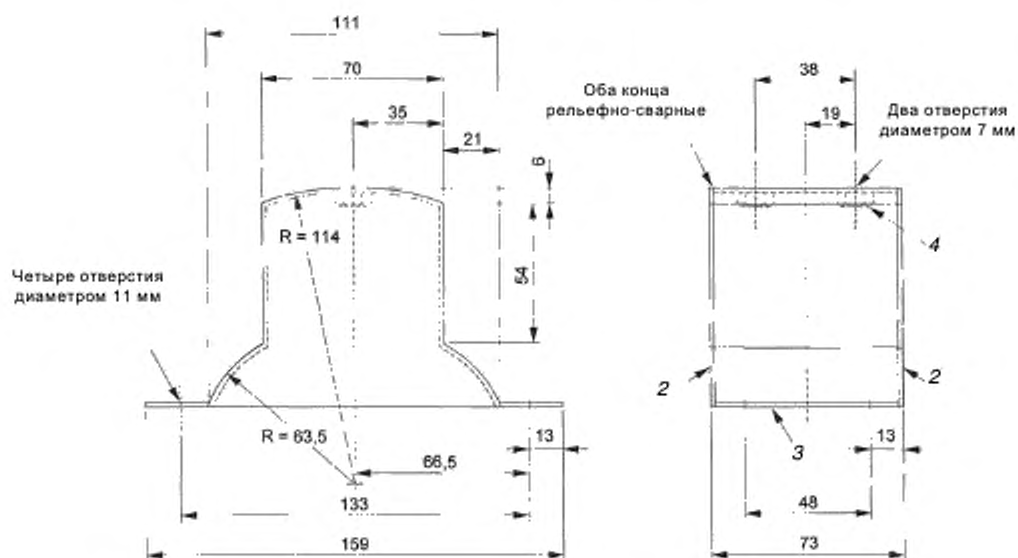
Рисунок В.2 — Нешаблонная обмотка, установленная на испытательную арматуру
