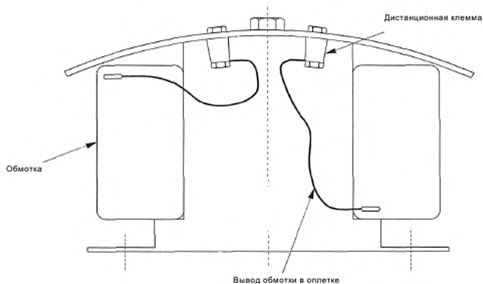
Рисунок В.6 — Измеряемая намотанная обмотка, установленная на испытательную арматуру
