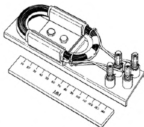
Рисунок А.2 — Полностью собранная и обработанная электроизоляционным лаком модель
