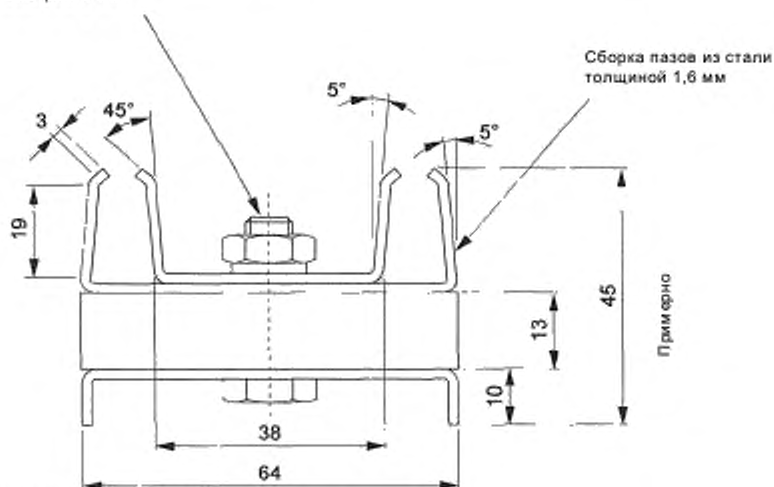
Рисунок А.3 — Производственный чертеж рамы модели
