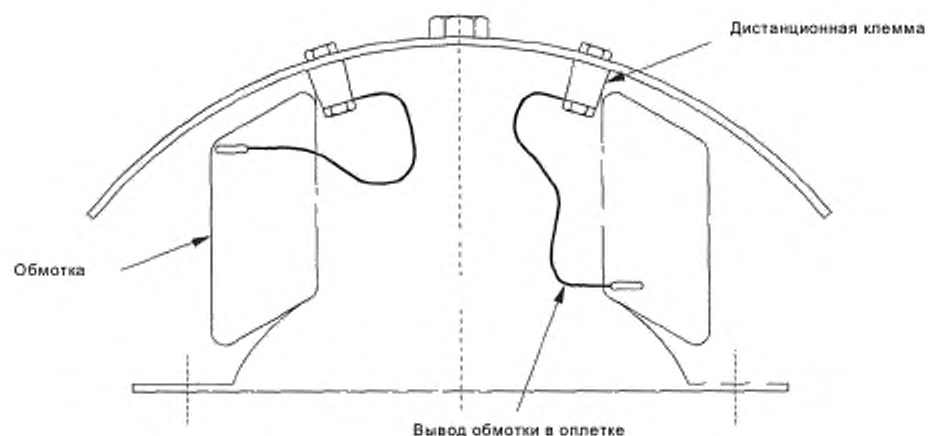
Рисунок В.2 — Нешаблонная обмотка, установленная на испытательную арматуру
