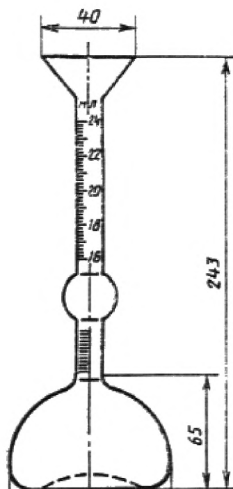
Рисунок 1 — Прибор Ле-Шателье
