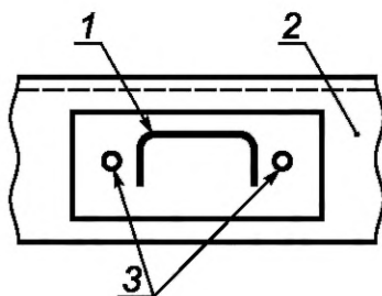
1 — кронштейн; 2 — лонжерон рамы; 3 — болты крепления
