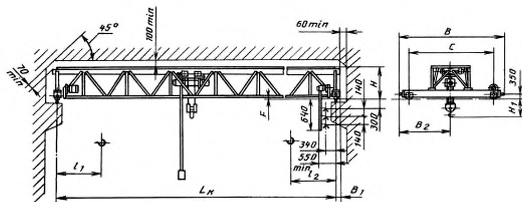
Кран типа 1 исполнения А для пролетов от 19,5 до 28,5 м
